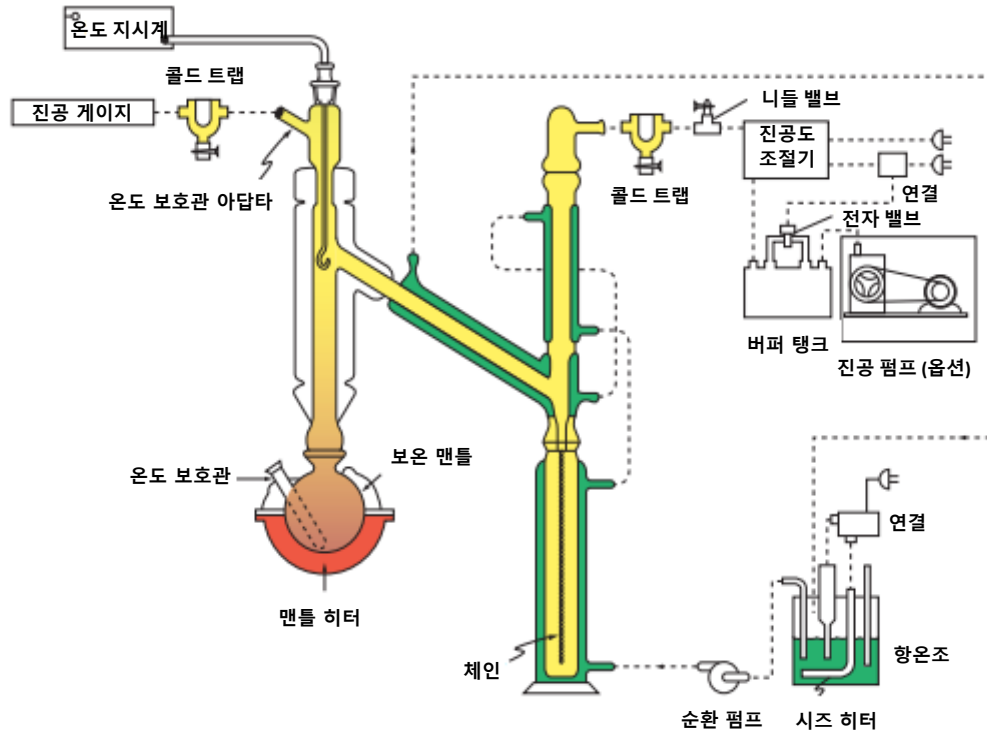
석유 제품 감압 증류장치
